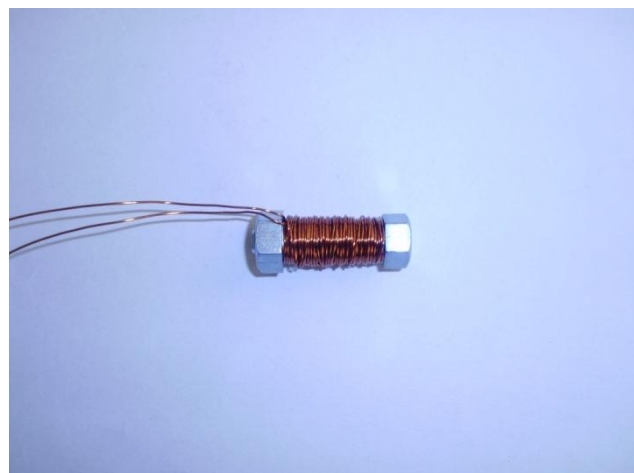
ボルトに紙を巻いた後，エナメル線を巻く。巻きはじめと終わりはエナメル線を長めに残しておいた方がよい。
